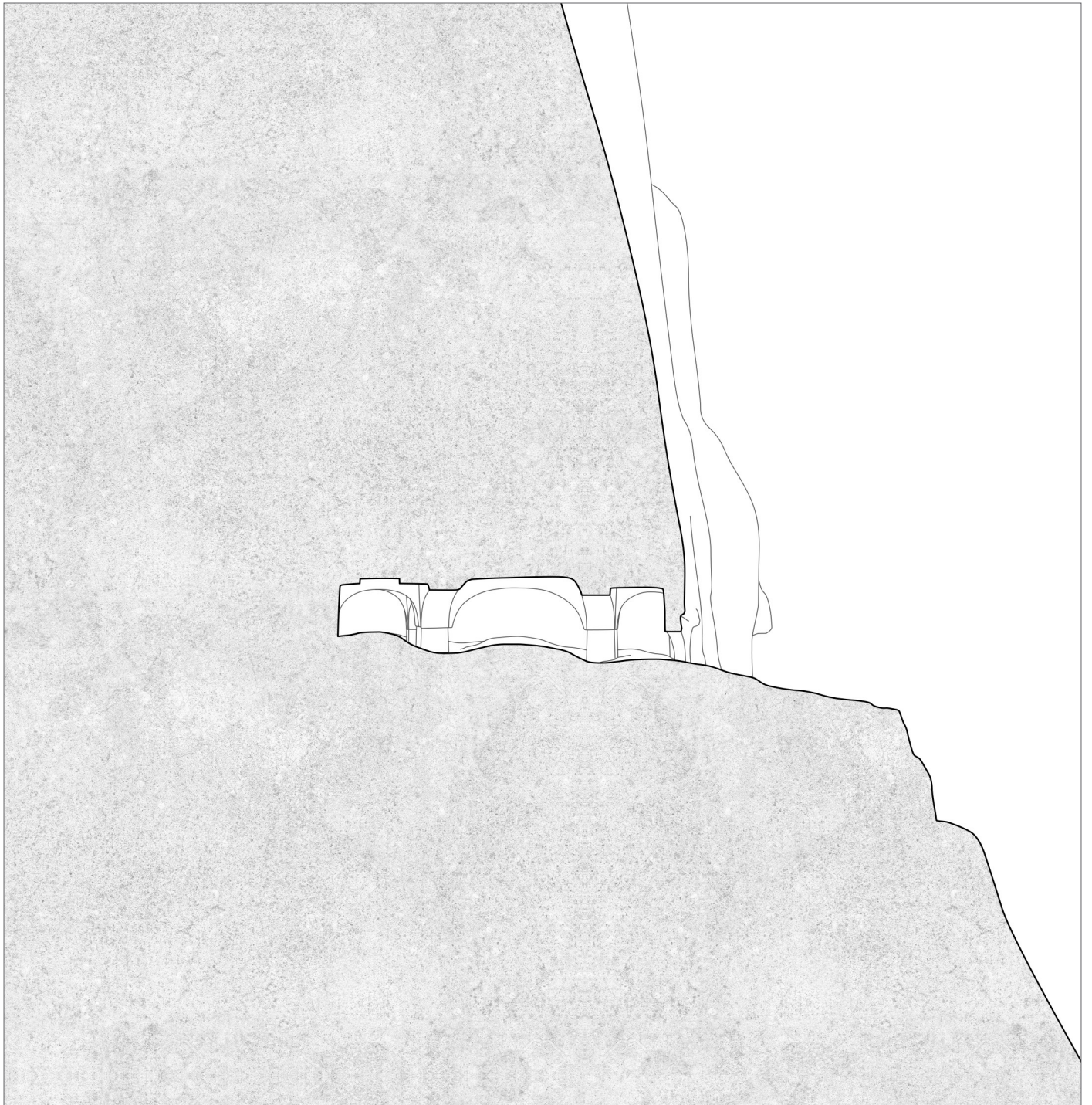
Medhane Alem Wäbrä Amba Section CC (2016)
